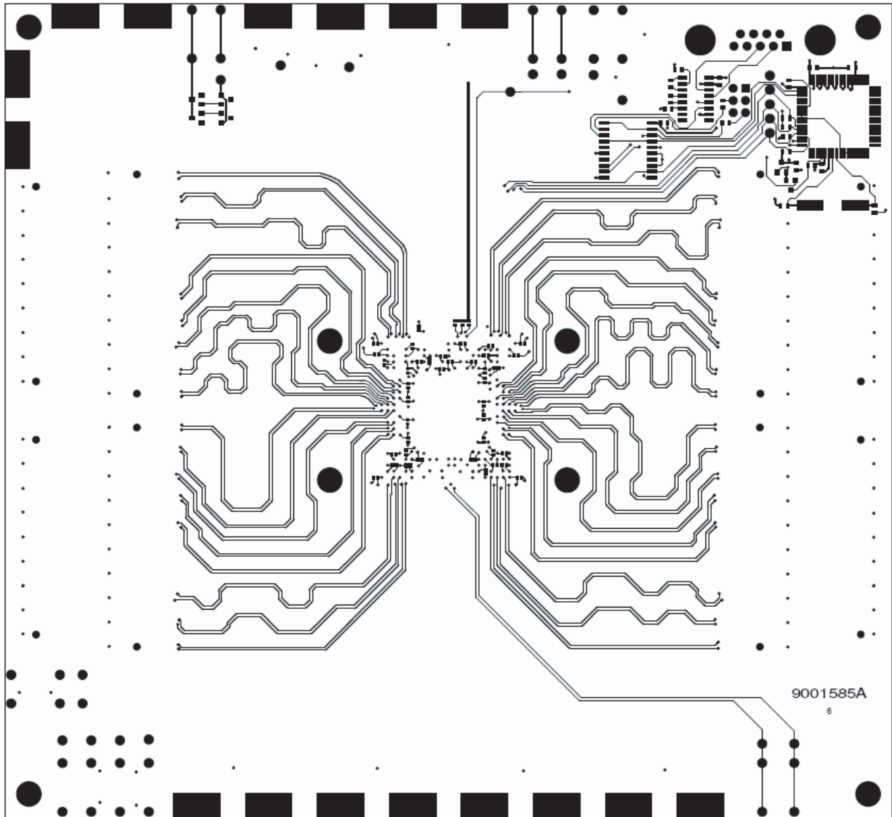
Figure 7-6. Bottom Layer
